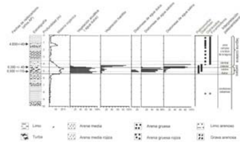
Figura 3. Secuencia Kino (KI), Sonora, resumen de datos de polen, diatomeas, ostrácodos y foraminíferos e interpretación paleoambiental.
