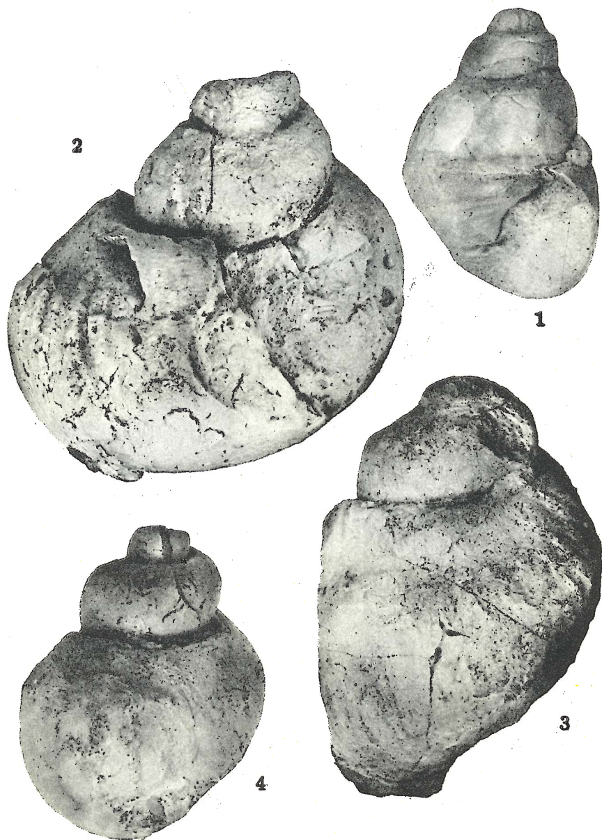
GASTEROPODOS DEL JURASICO SUPERIOR
